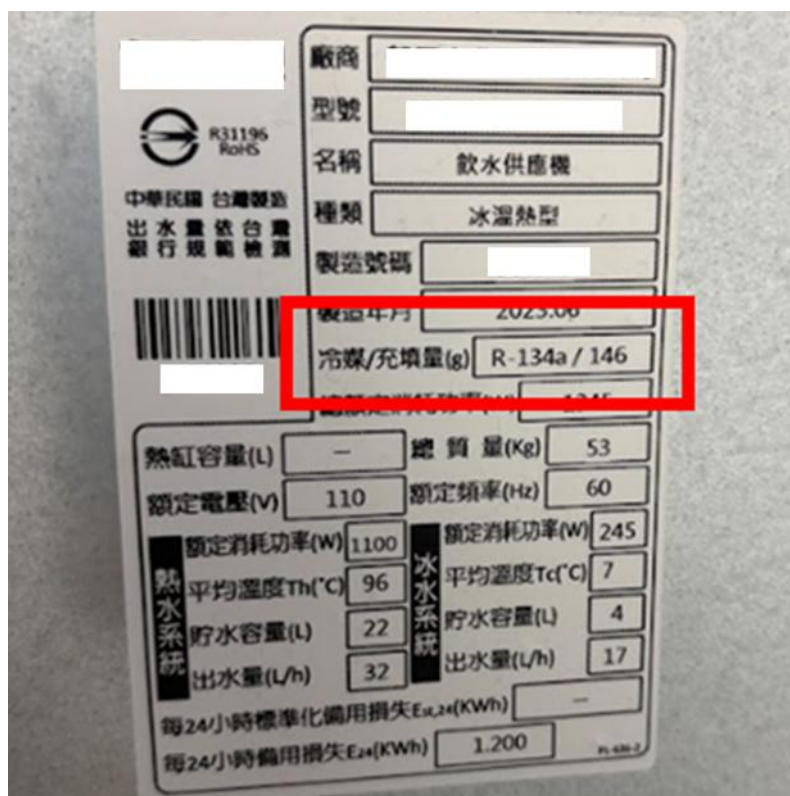
圖 2-10、冰溫熱飲水機銘牌範例
