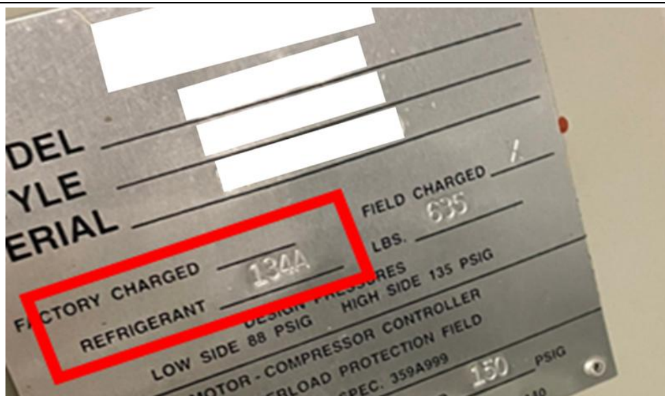
圖 2-9、冰水主機銘牌範例
